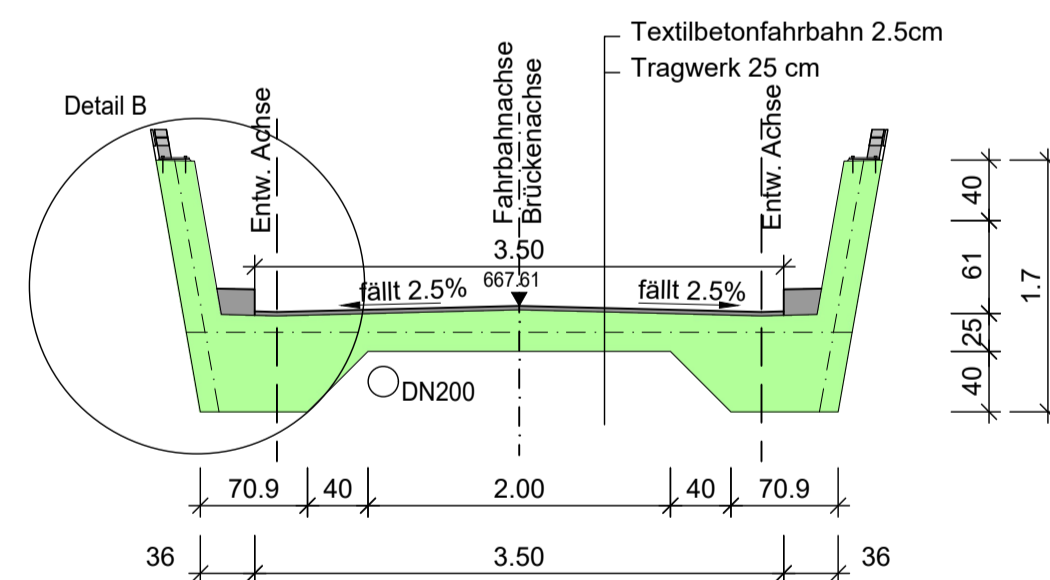
Schnitt B-B M 1:50
