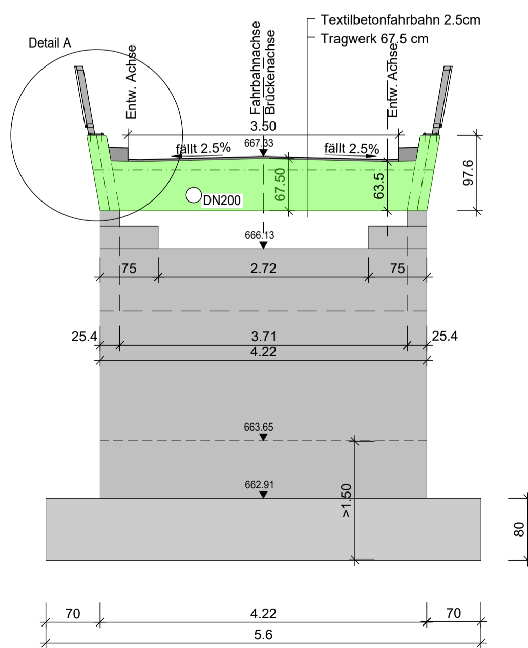
Schnitt A-A M 1:50
